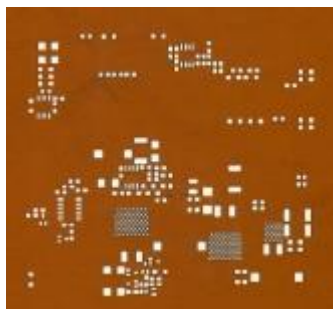
SMD-masky z polyimidu Kapton
